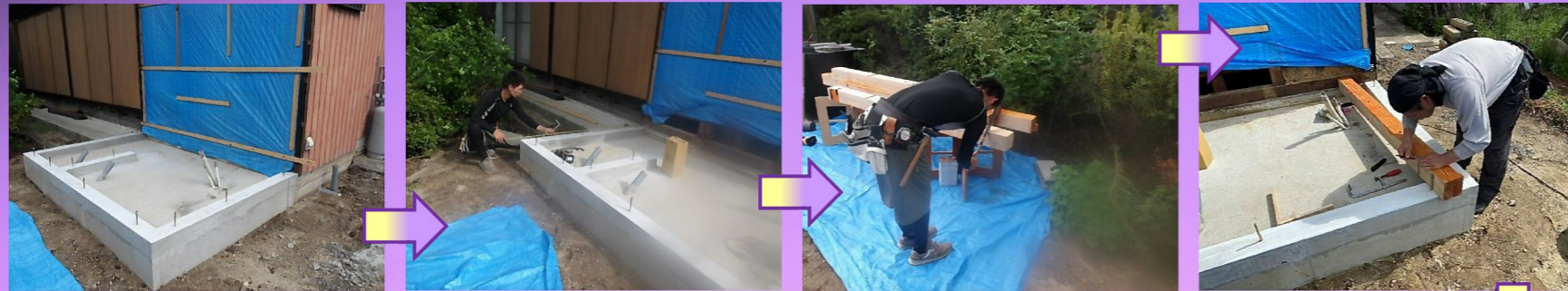
基礎の養生期間が終わり、土台敷きを行います。
