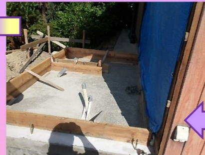
型枠をばらして立ち上がり部の角をサンダーで削ってを整え、基礎周りに一時撤去していた土を戻して工事完了です。
