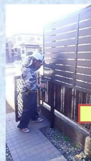
既設の木製フェンスを撤去し、アルミフェンスを組み上げていきます。
